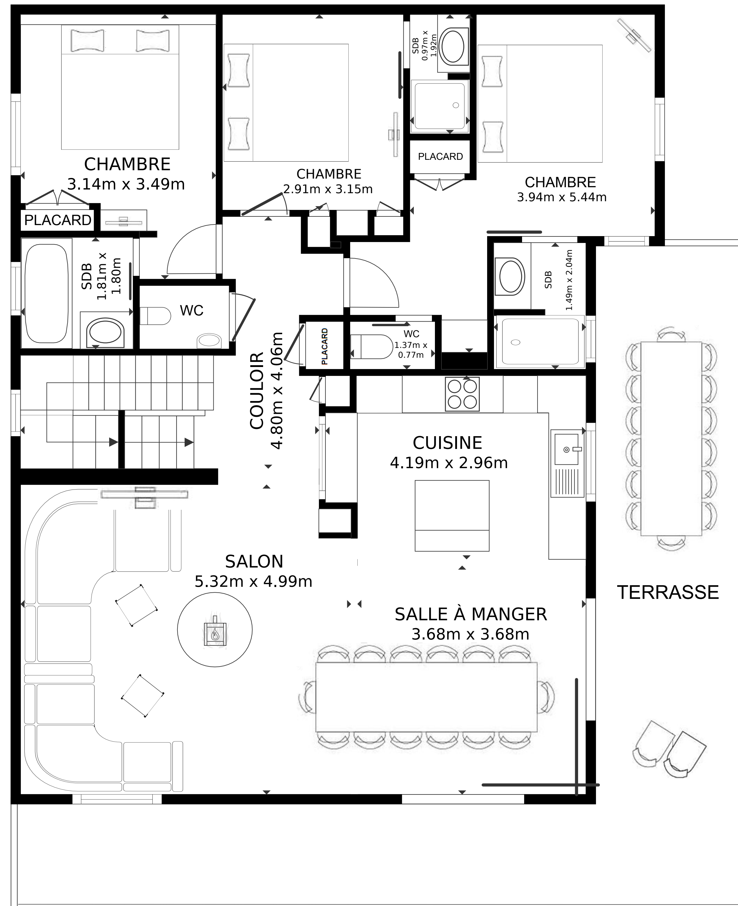
ÉTAGE 1
